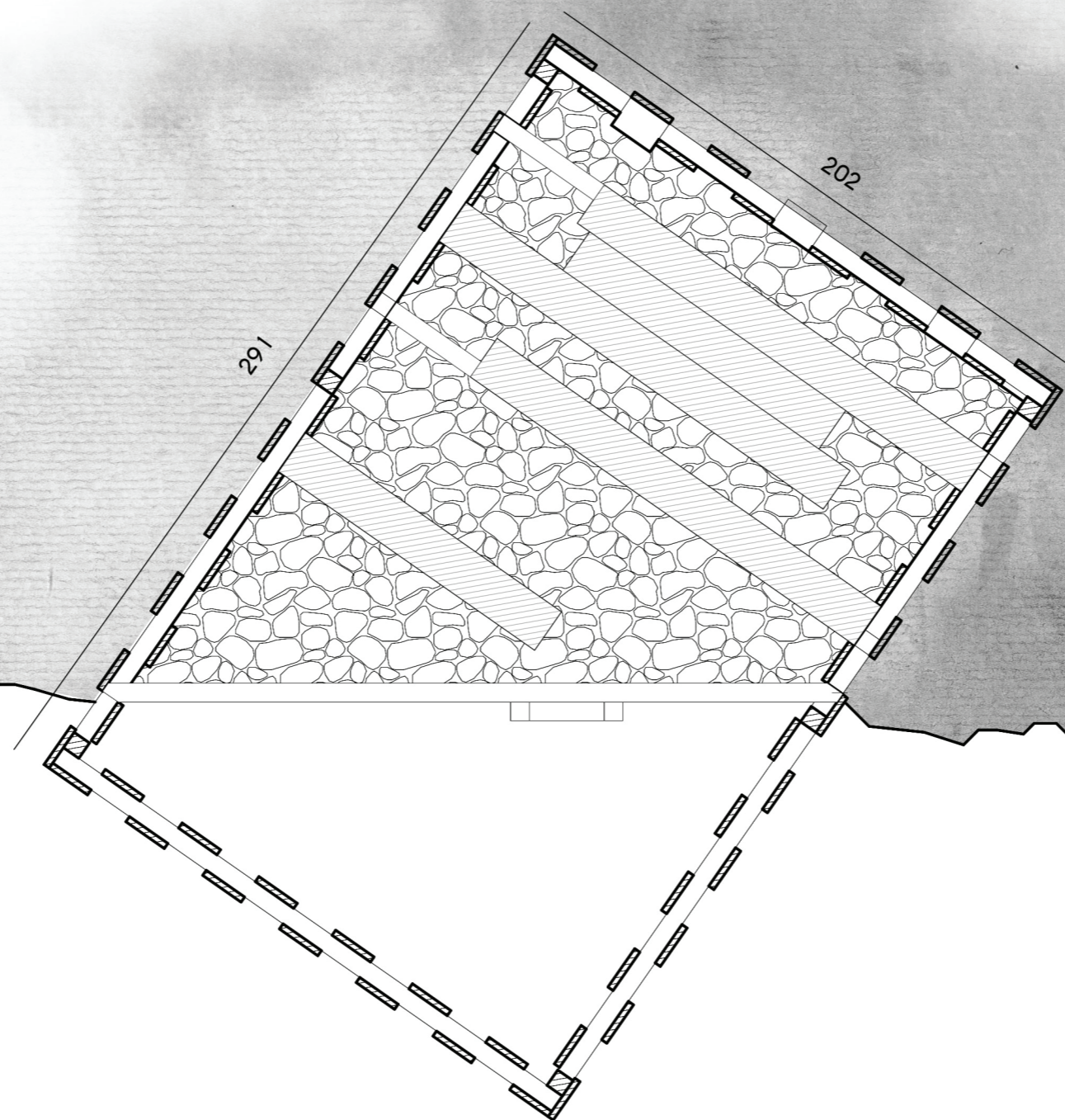
PLAN DE LA CABANE 1/20
